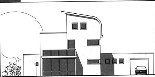
aanzicht straatgevel
