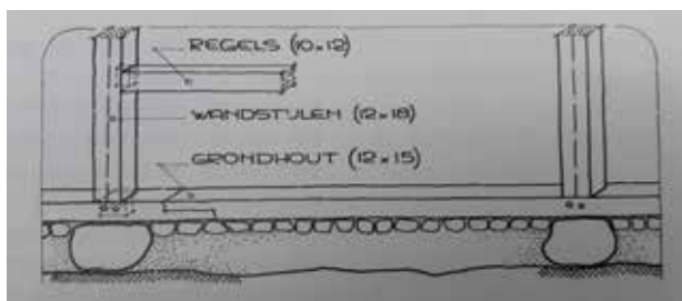
Het grondhout gedragen door veldkeien (uit: De bouw van een Twentse boerderij 1984)
